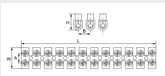
Габаритные размеры
